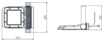
【金具寸法】 ※共通
