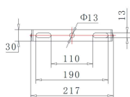
【金具寸法】 ※共通
