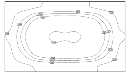
【配光図】 ※水銀灯400Wの場合
