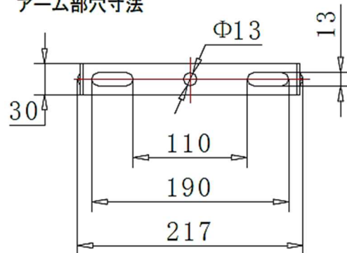
アーム部穴寸法
