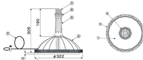
【B3B-150/180/200-150D】
