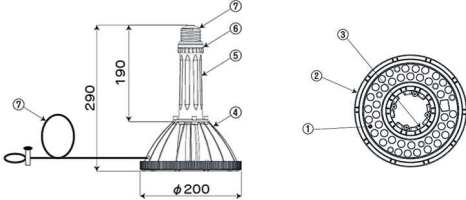
【金具寸法】
