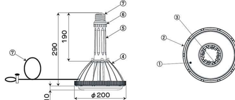
【B1B-40/50/60/80-150D】
