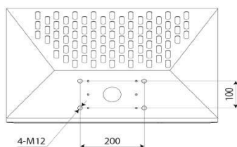
姿図
